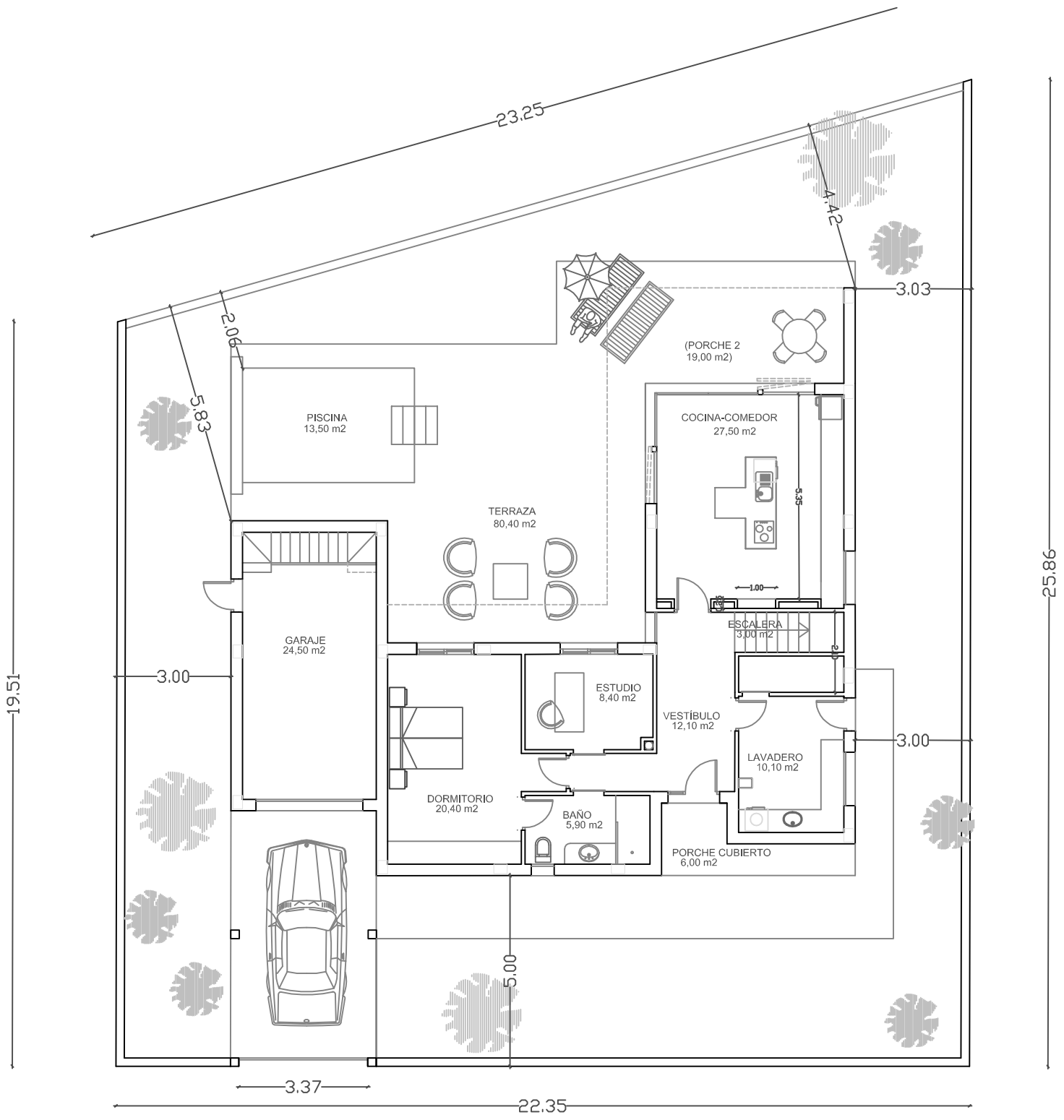
PLANTA BAJA
